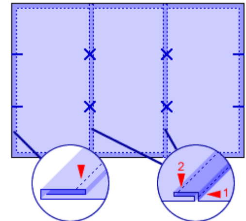
Figura 2. Detalle de las costuras
