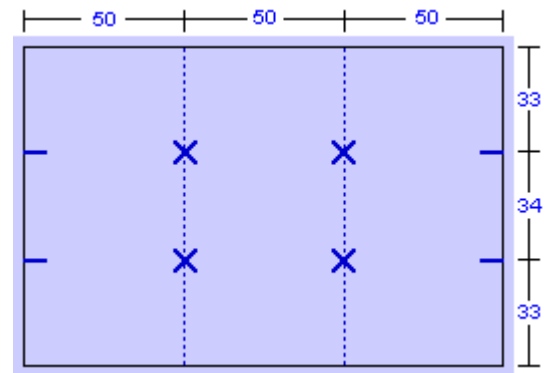
Figura 1. pieza de tela de 150x100cm (con algo de margen)
