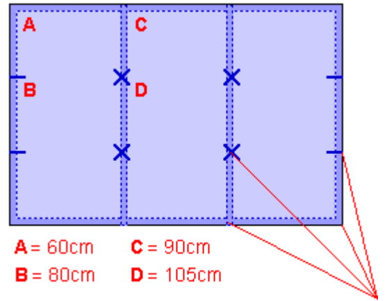
Figura 3. La brida del moco, con sus medidas
