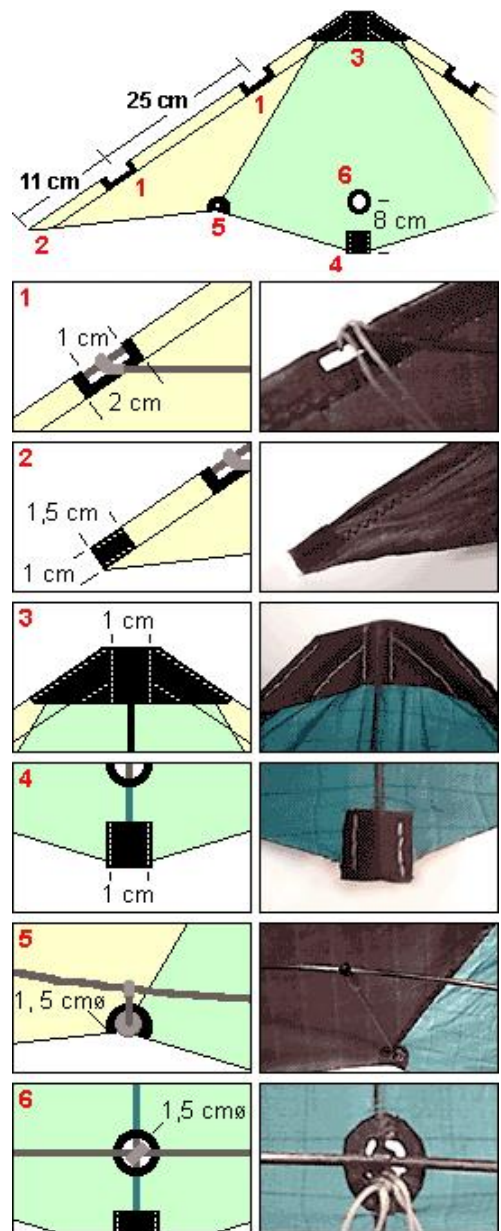
Figura 2. detalles de la Kitty
